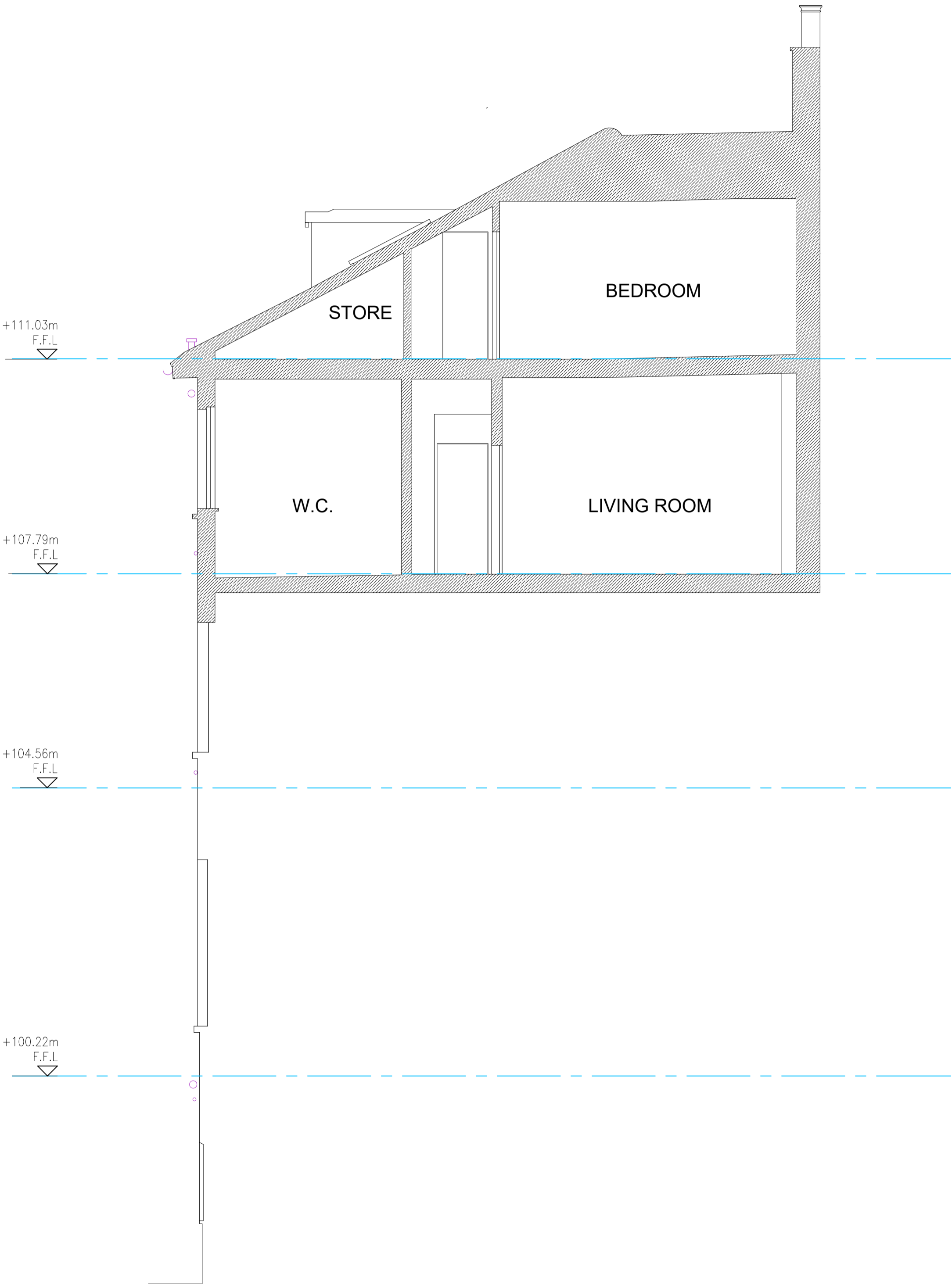
01 SECTION 1 SC-006 1:50@A1 / 1:100@A3
