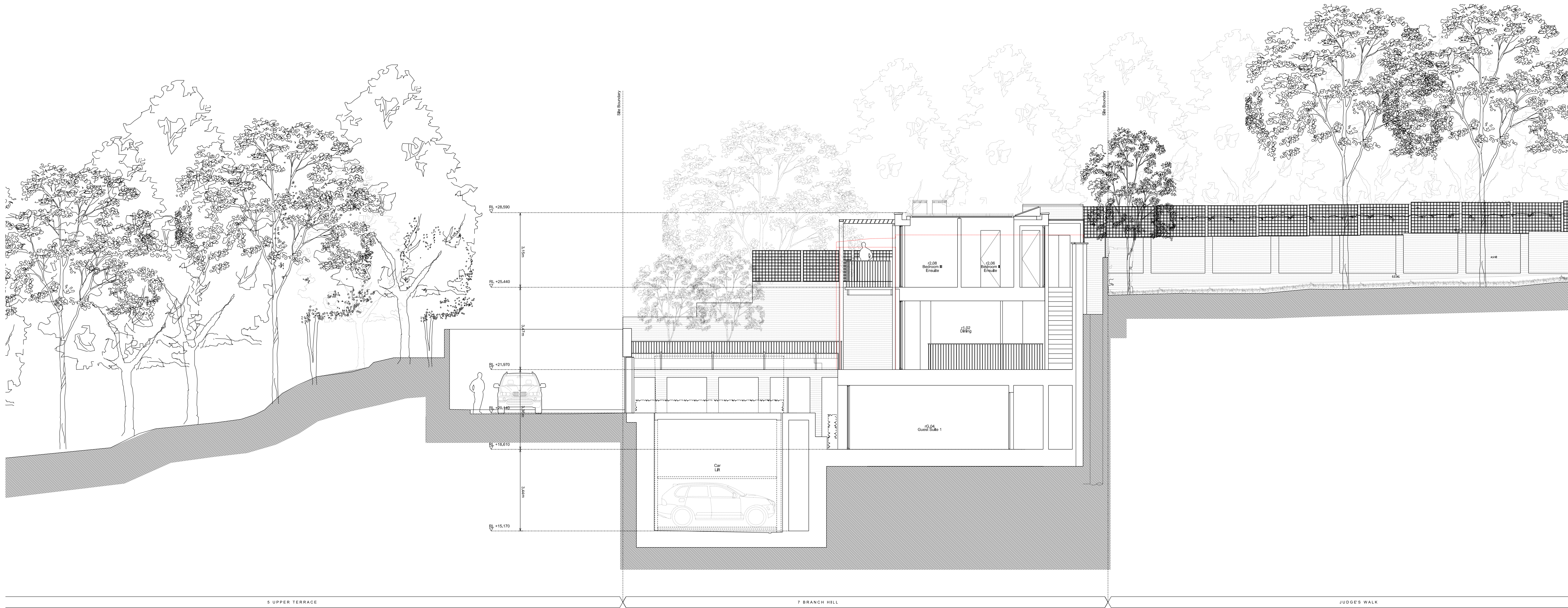
Existing Section DD
