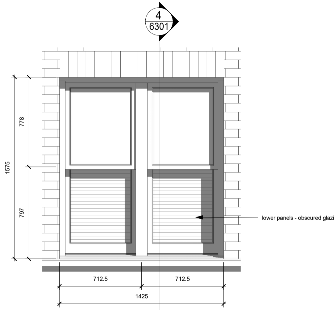
3 Win-04 DET_Elevation 1 : 20
