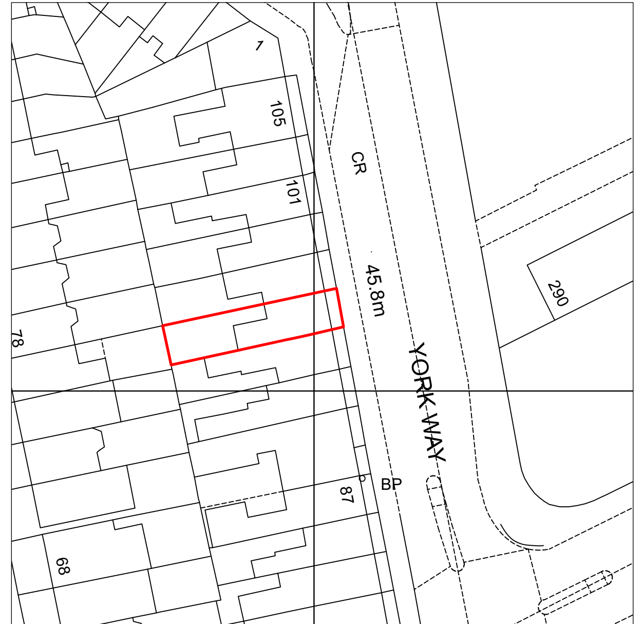
2 BLOCK PLAN Scale: 1:500 @ A3
