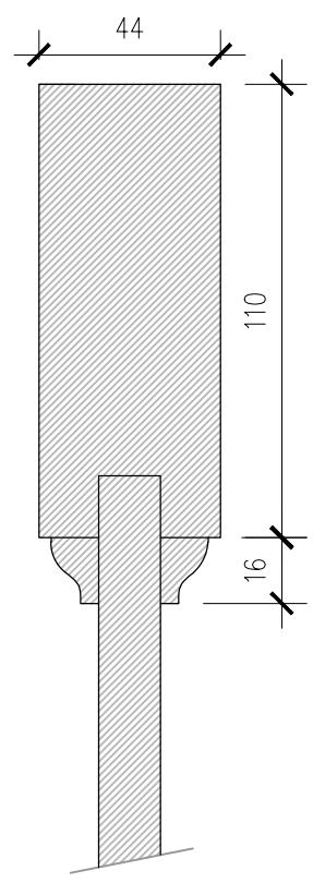
DOOR TYPE 03/03a PROFILE DETAIL HIERARCHY 3 REGENCY FOUR PANEL DOOR SCALE - 1:2
