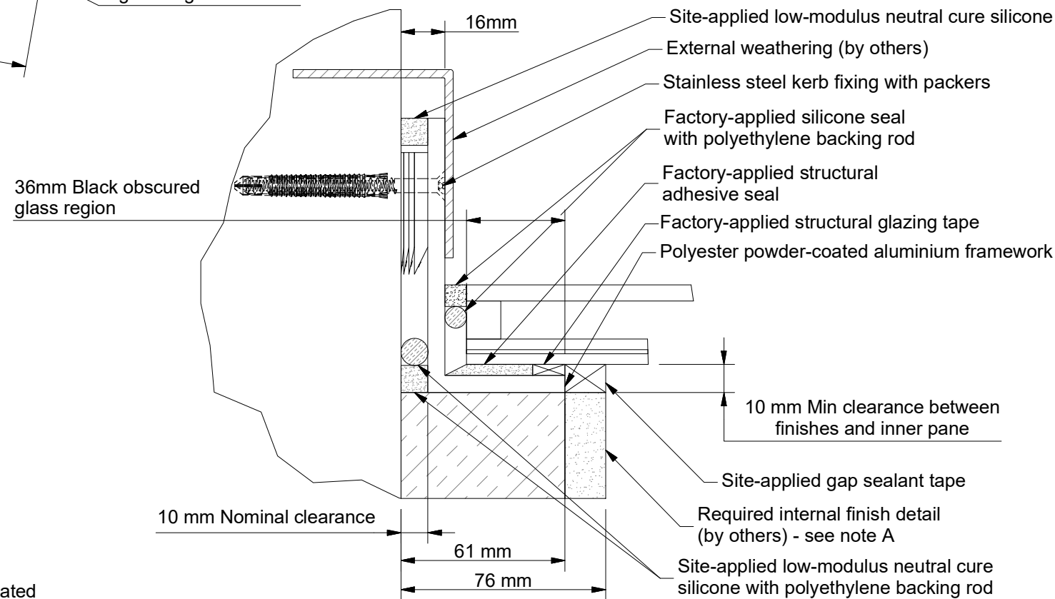
Detail D ( Scale 1:2 )
