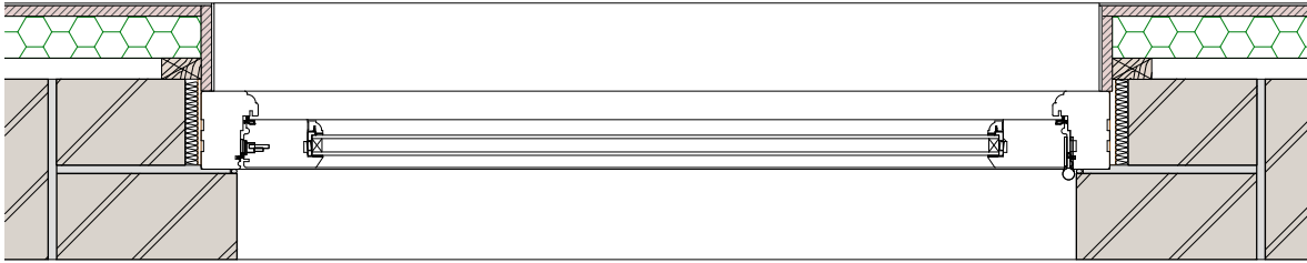
2 Plan 1:10
