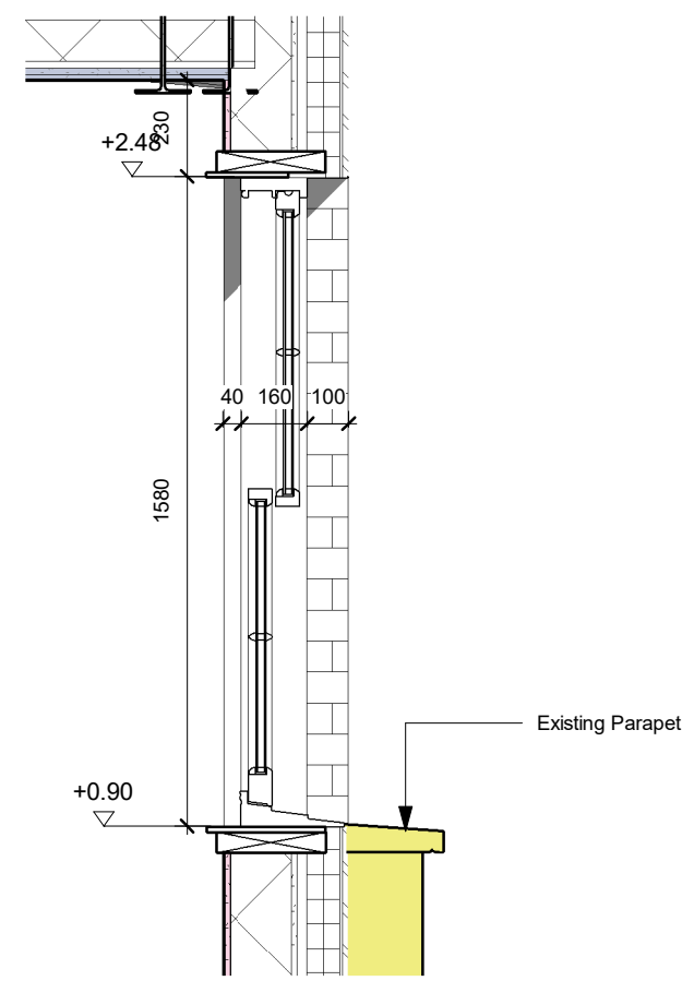
4 Win-04 DET_Section 1 : 20
