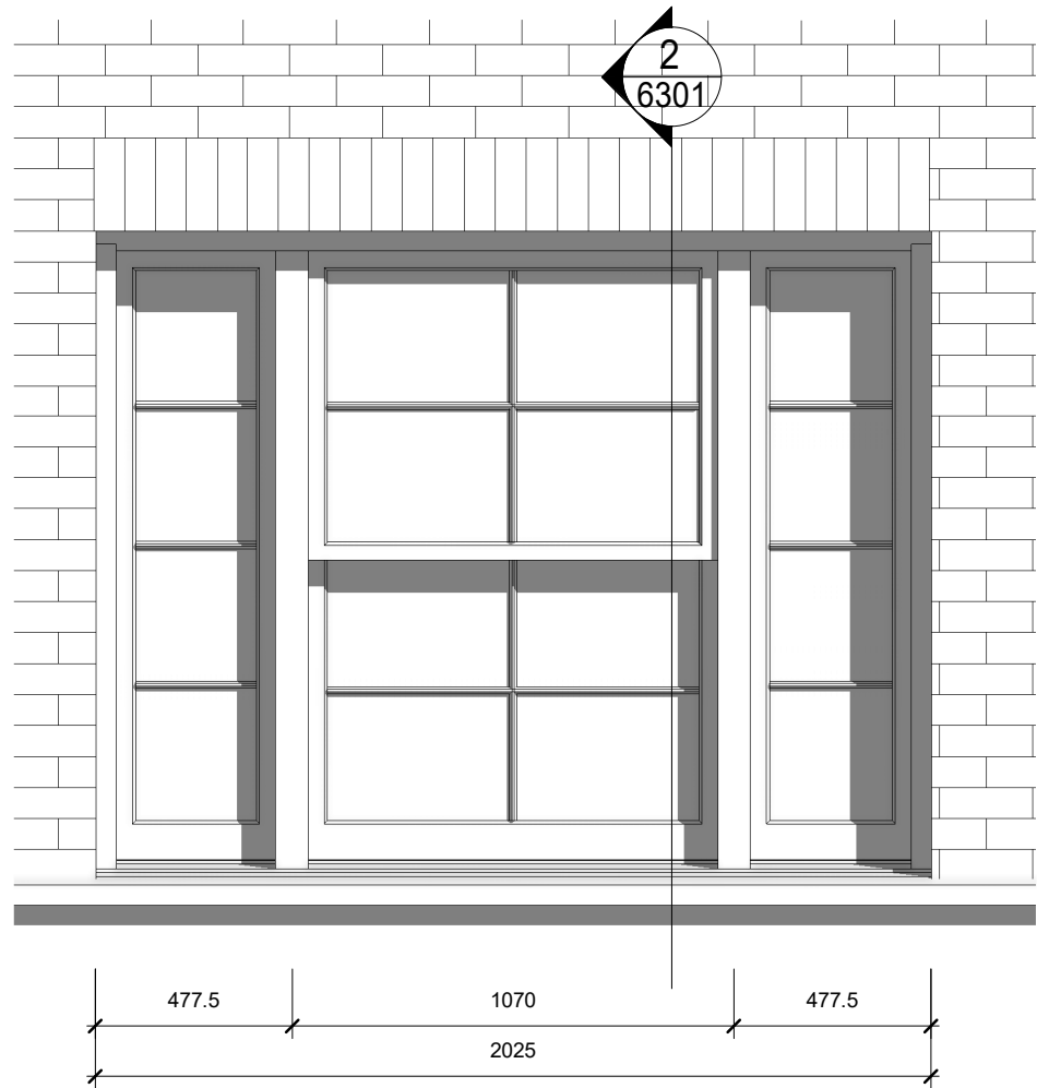
1 Win-01,02,03,05 DET_Elevation 1 : 20
