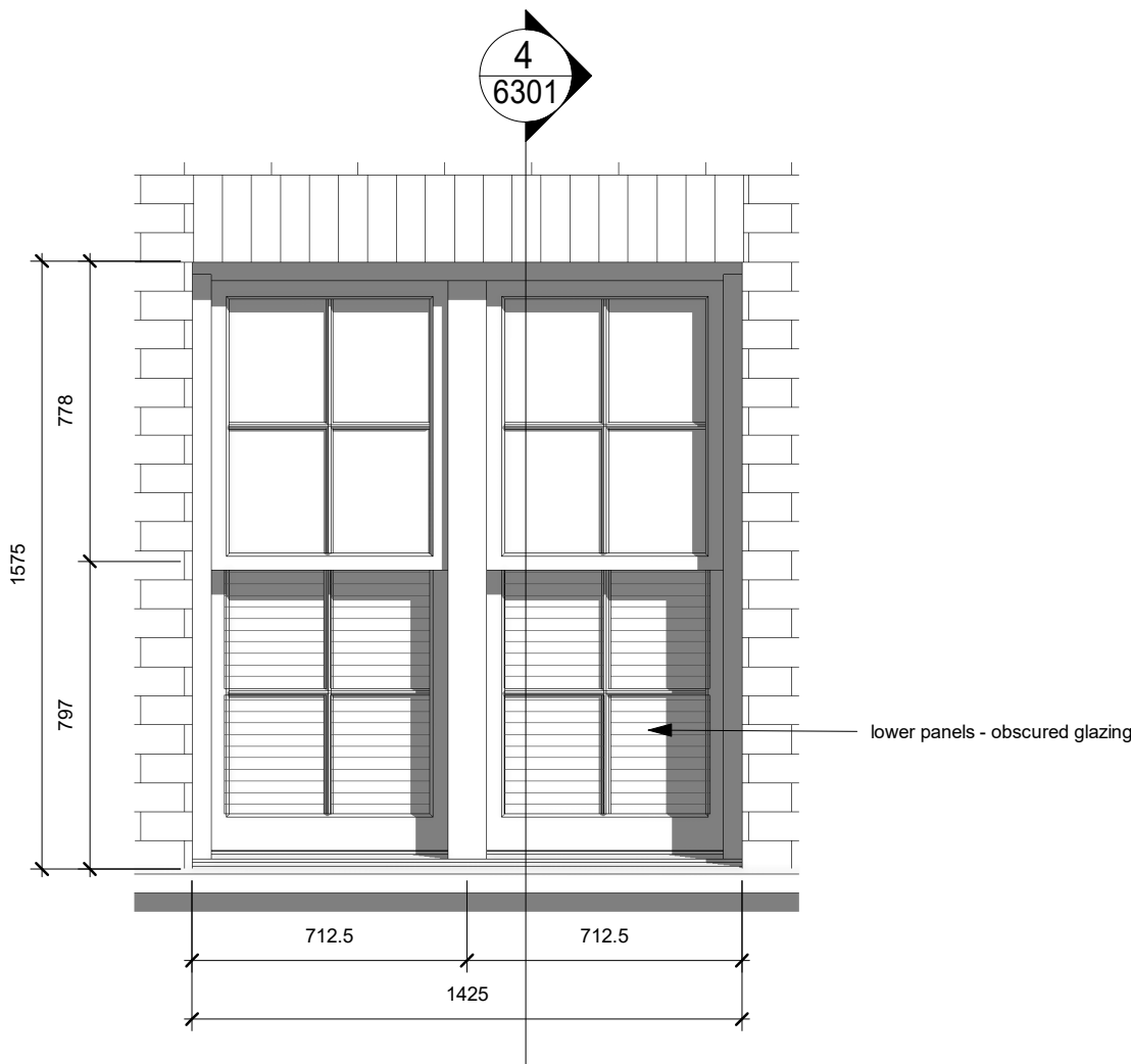
3 Win-04 DET_Elevation 1 : 20
