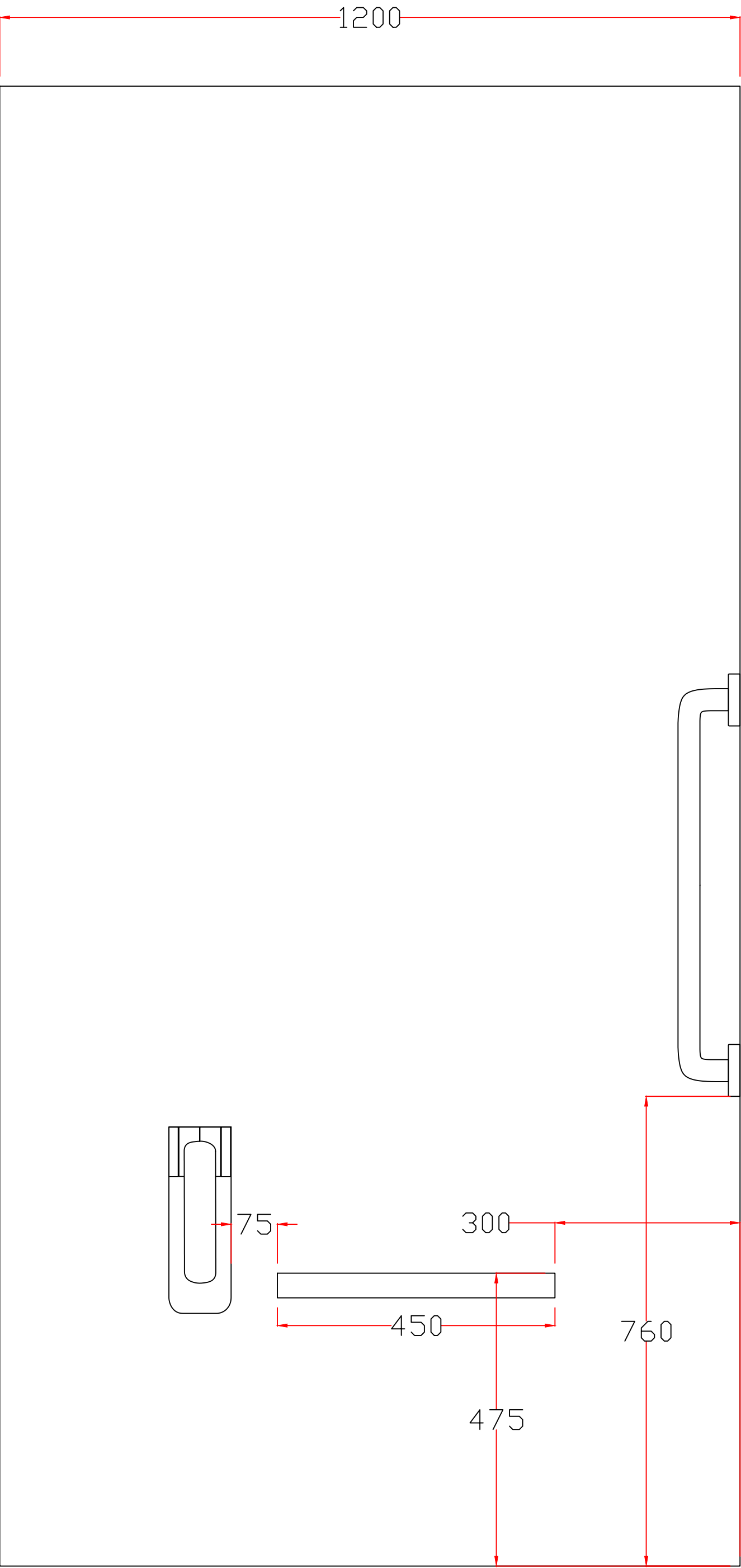
ELEVATION A-A
