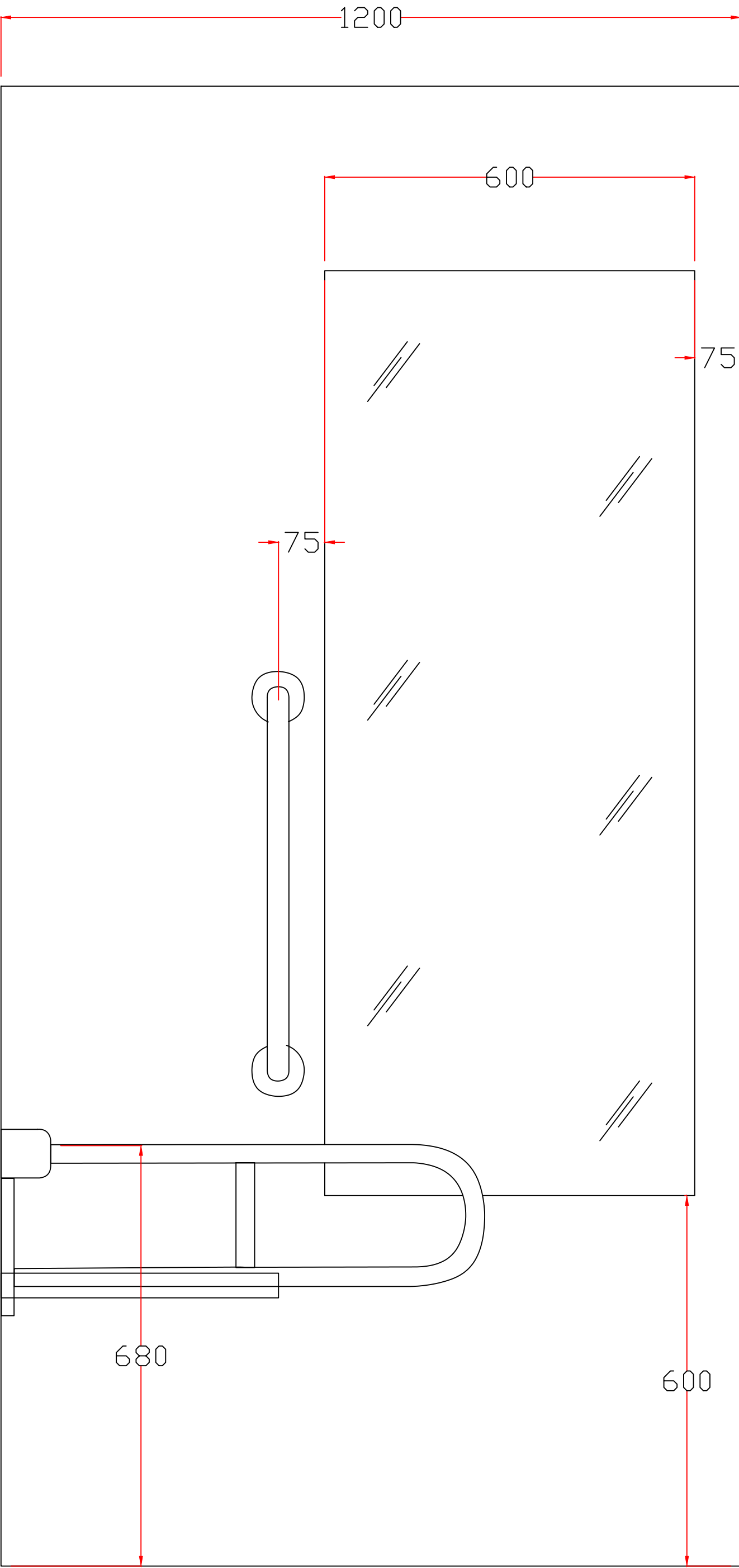
ELEVATION B-B
