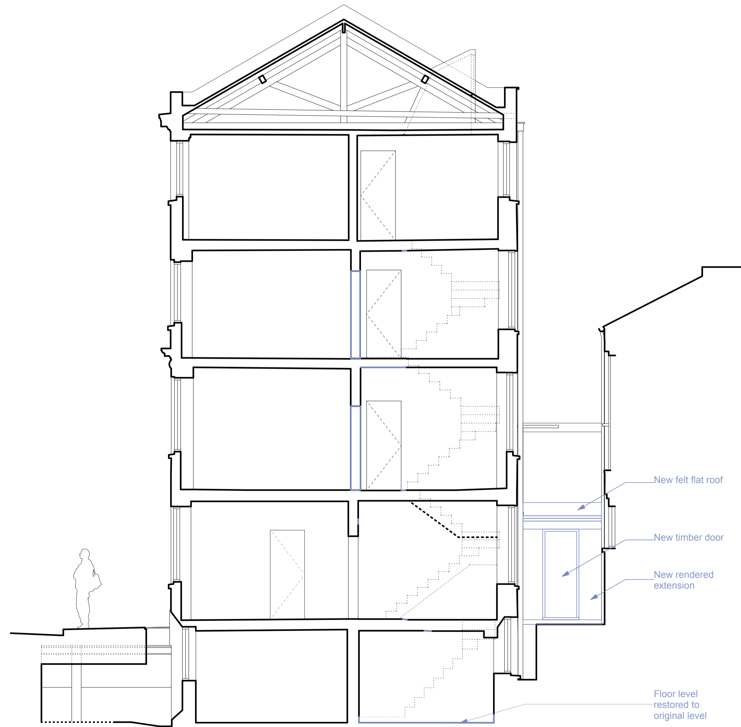
SECTION A-A
