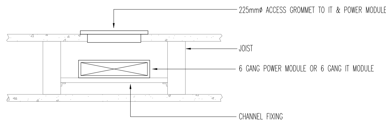
POWER/IT MODULE DETAIL (SCALE 1:10)
