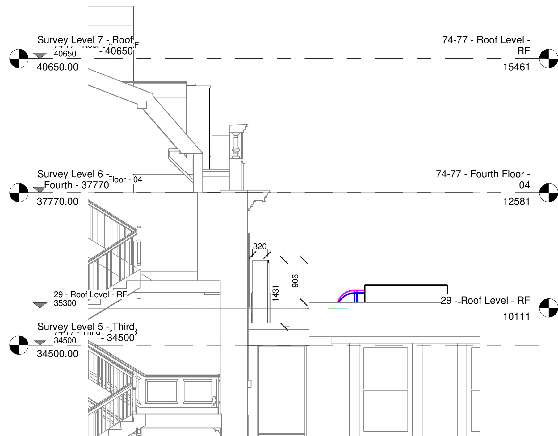
1 Section 2 - Option 2 1 : 50
