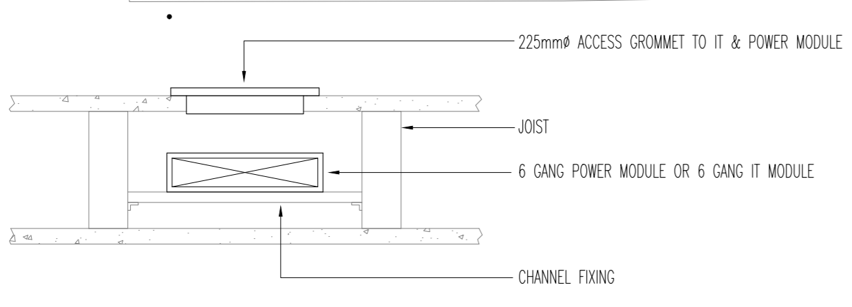
POWER/IT MODULE DETAIL (SCALE 1:10)
