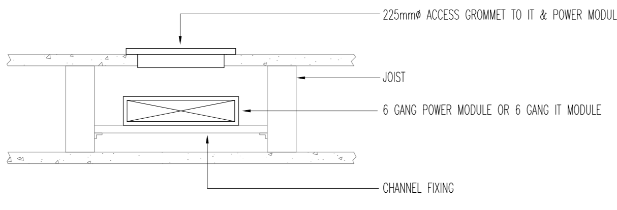
POWER/IT MODULE DETAIL (SCALE 1:10)
