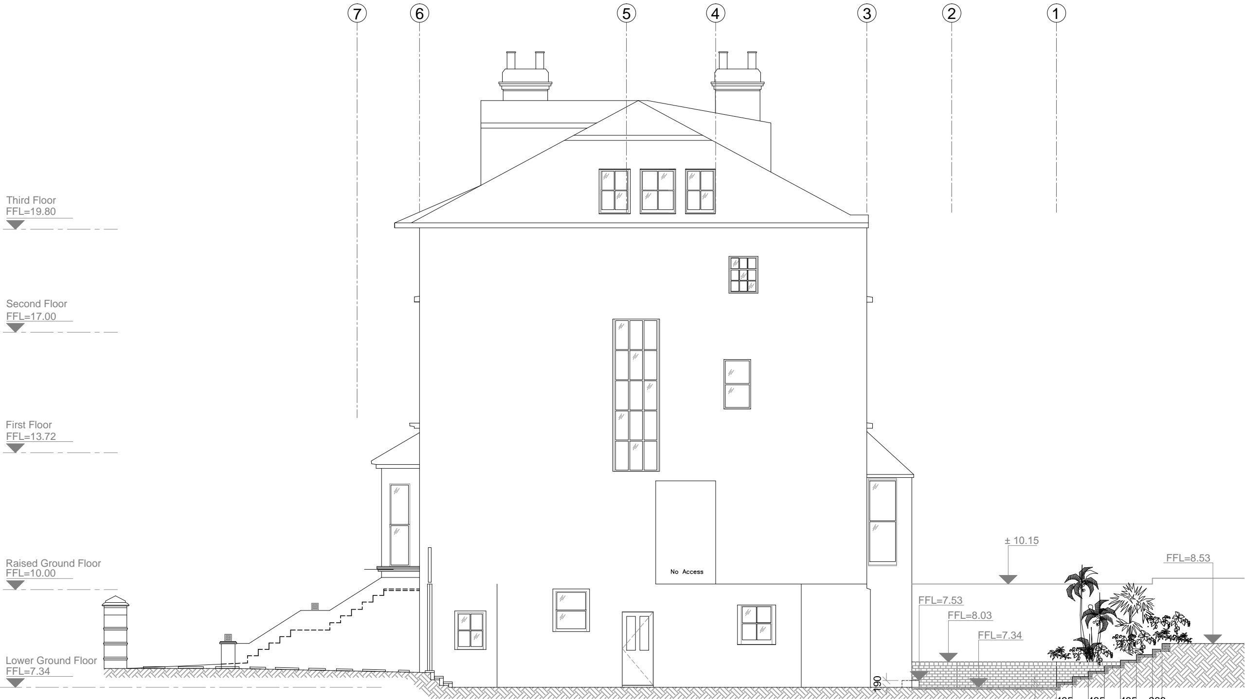
Existing SECTION C-C (1-2) SCALE: 1:100 on A3
