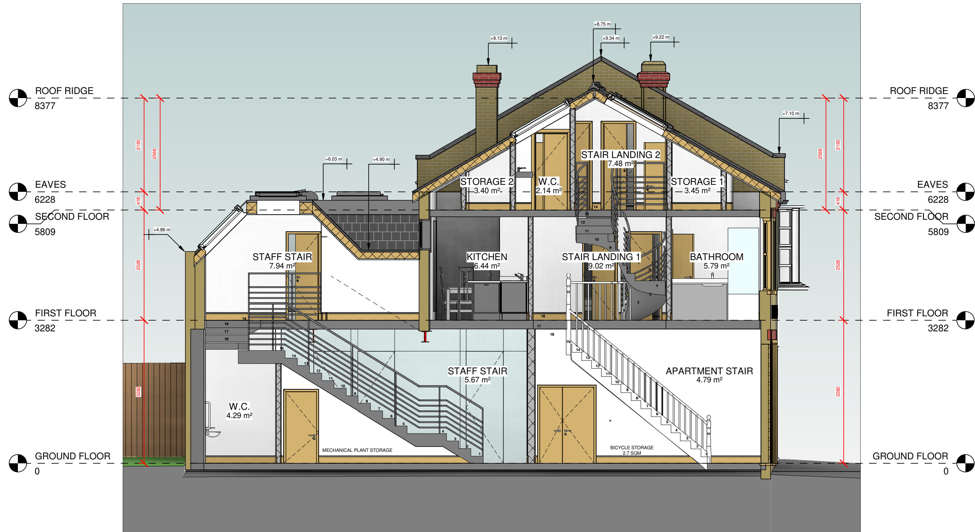
1 SECTION 1 1 : 50
