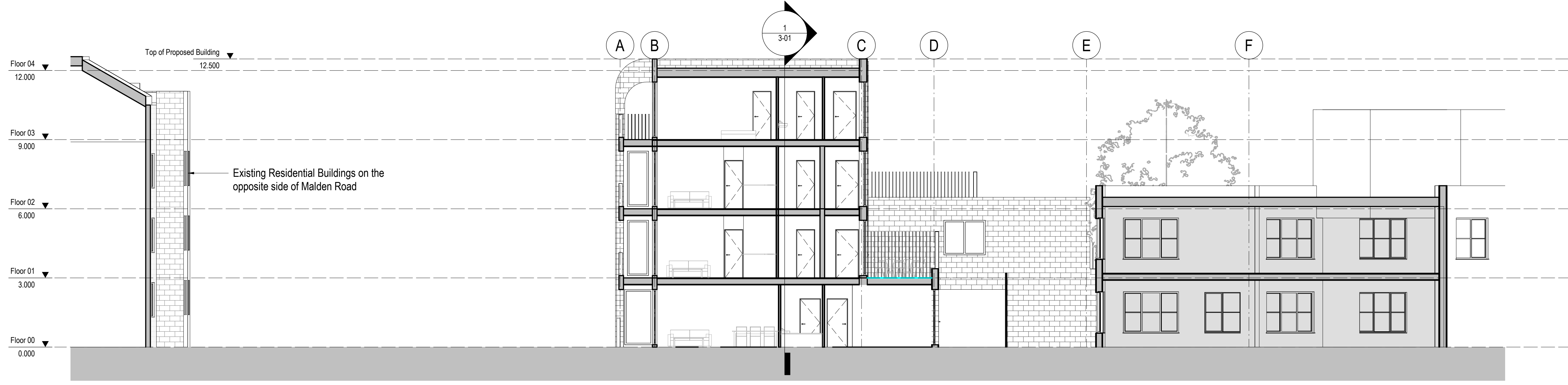
3 Section 3 1:100
