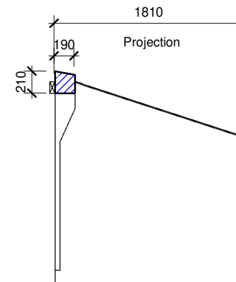
Awning box side section 1 : 50
