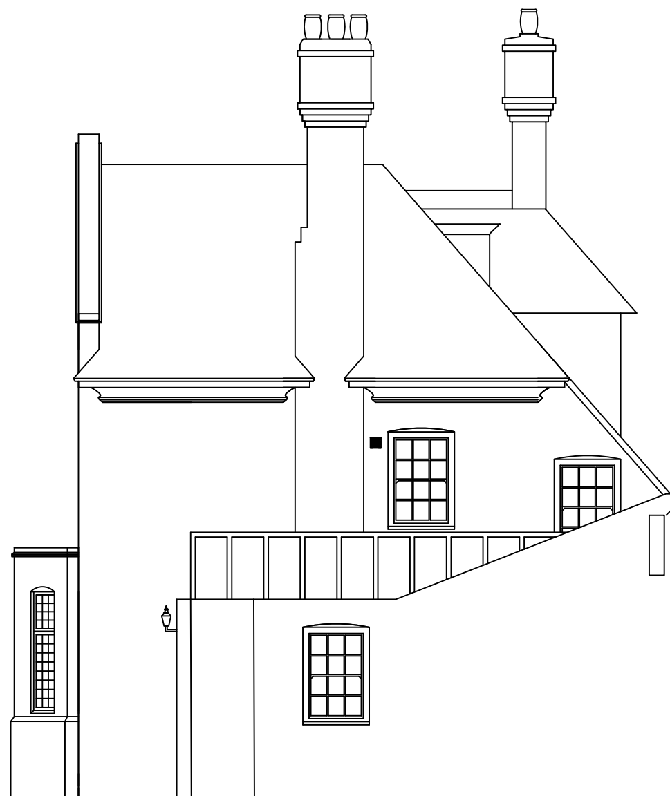
Existing Right Flank Elevation
