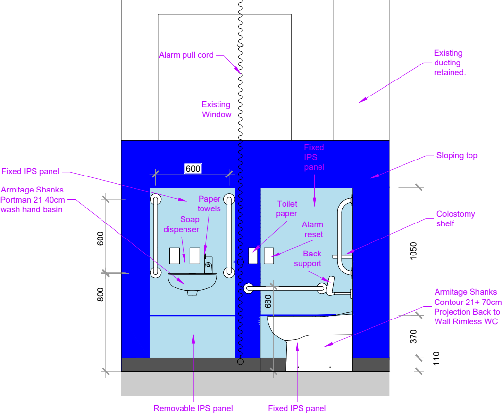
Elevation B.
