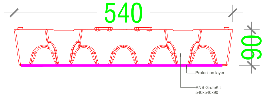
Section - ANS GrufeKit Scale - 1:5
