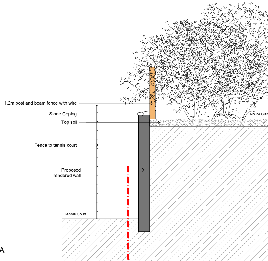
1 Elevation 1:100
