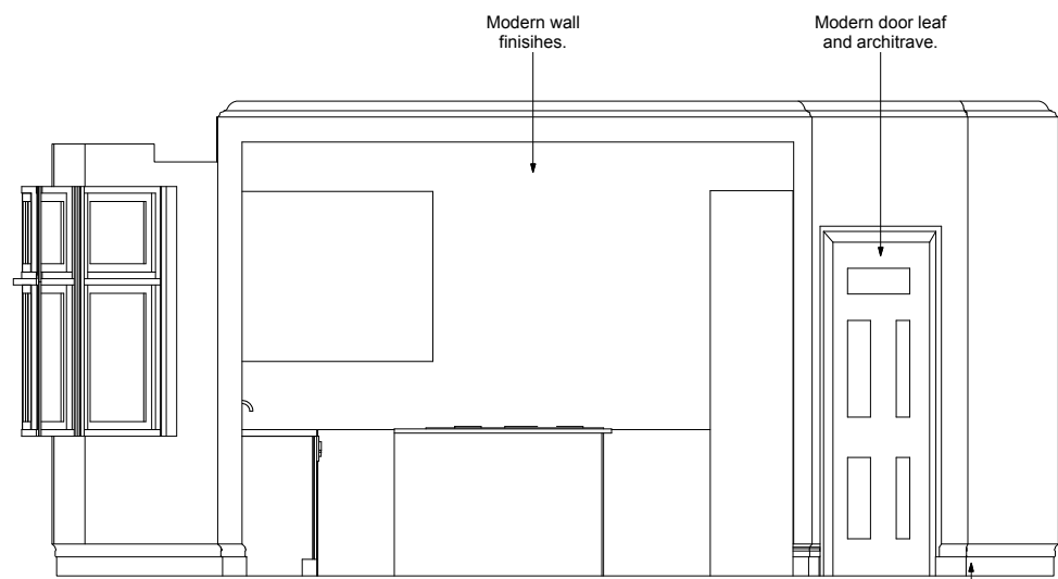
A Dining Room - Elevation A Scale: 1:50 @ A3
