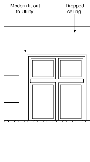
A Utility - Elevation A Scale: 1:50 @ A3
