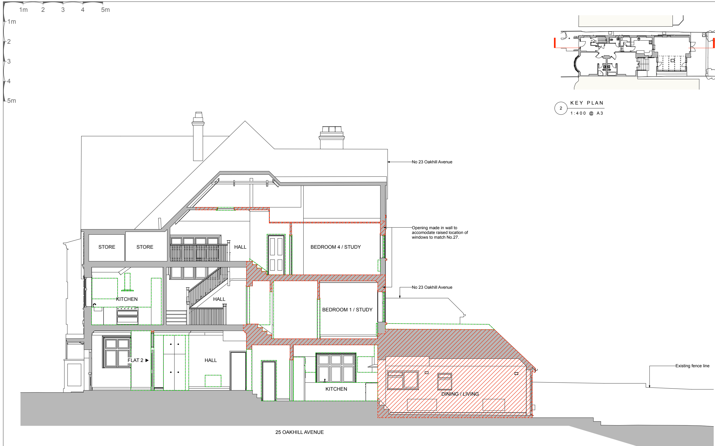
BB EXISTING SECTION BB 1:100 @ A3
