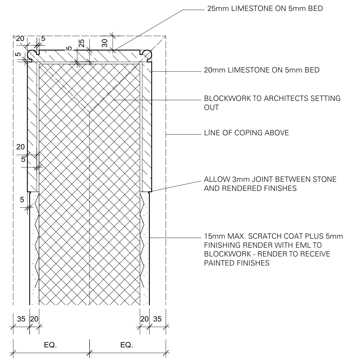
5 PORCH QUOIN - PLAN Scale: 1:5
