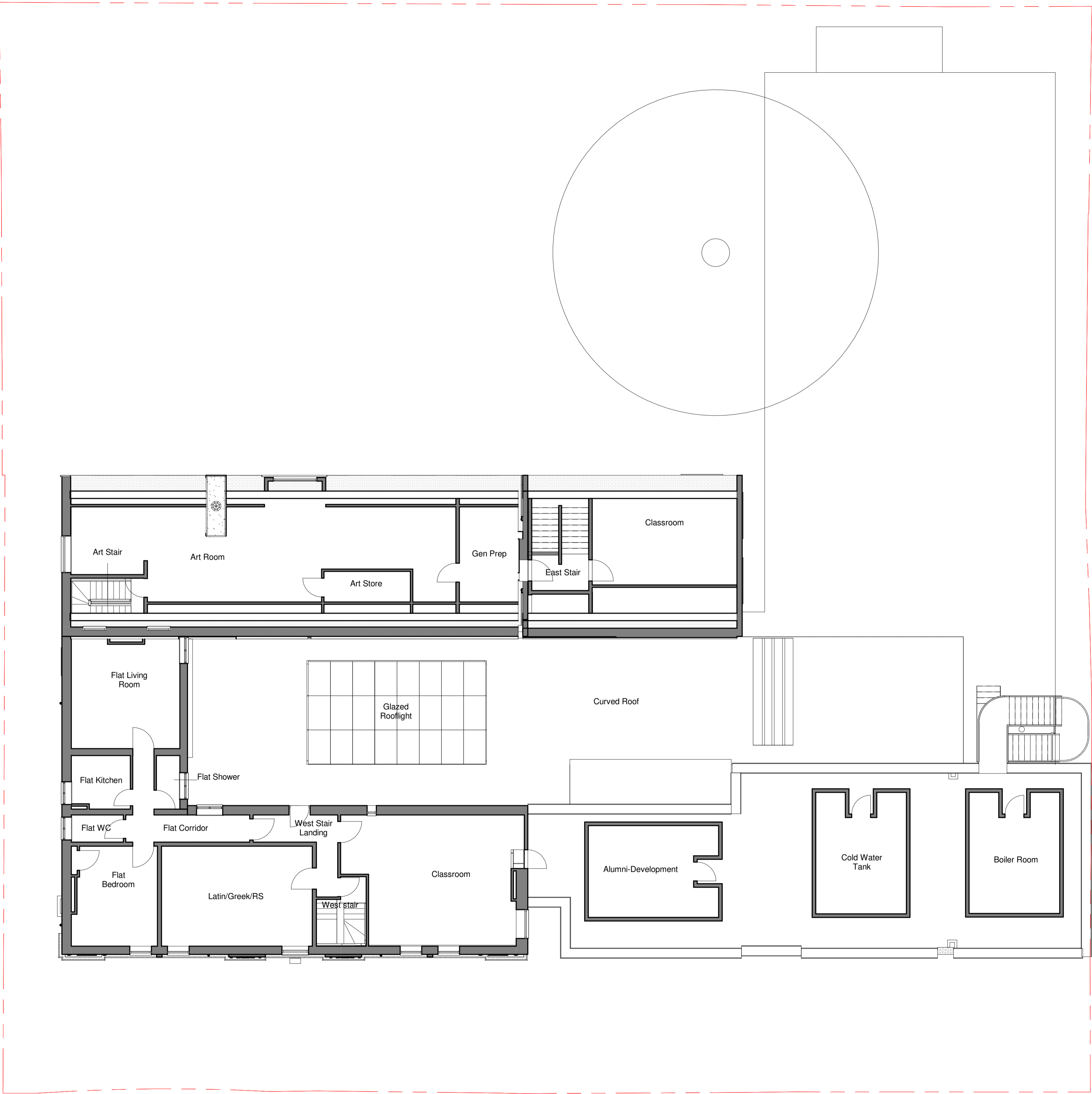
EXISTING GA - LEVEL 02 1 : 100
