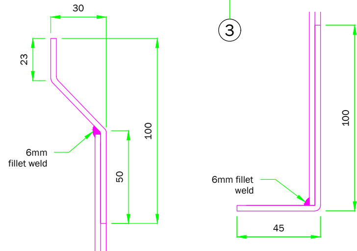
A Section A-A scale 1:2
