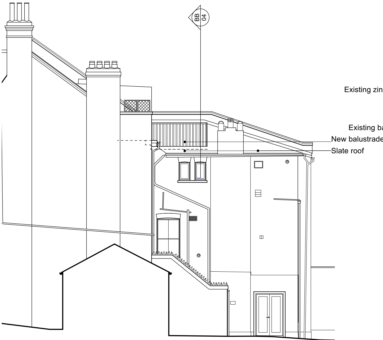
01 005 ELEVATION SIDE
