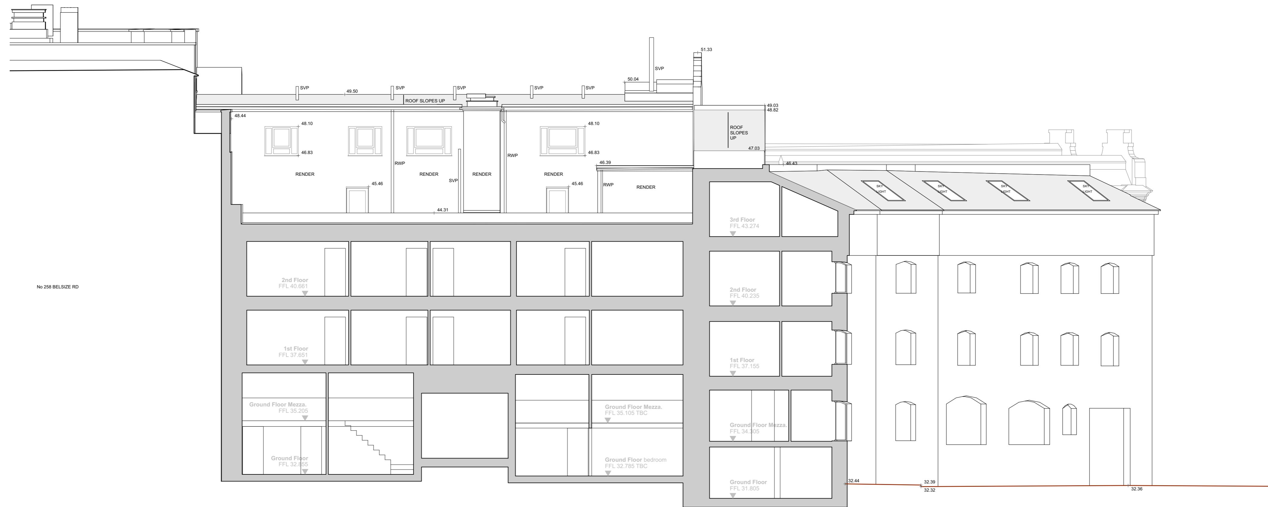
SECTION D-D
