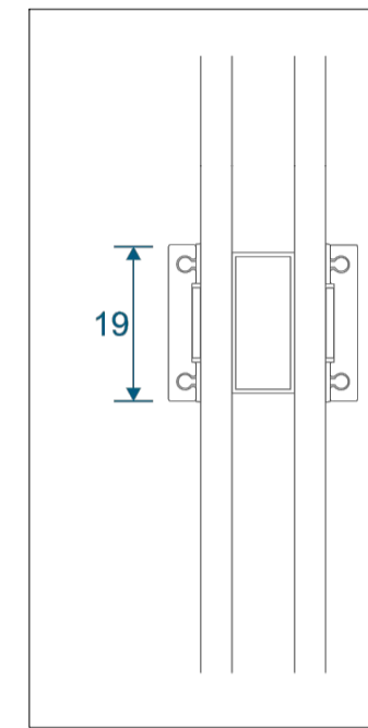
Astragal bar
