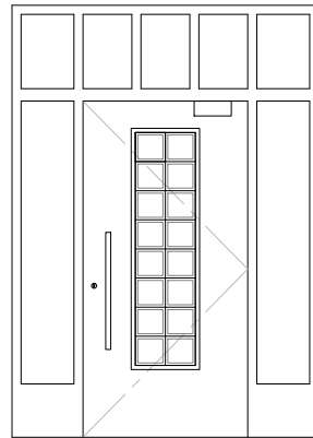
Existing 01 / C04
