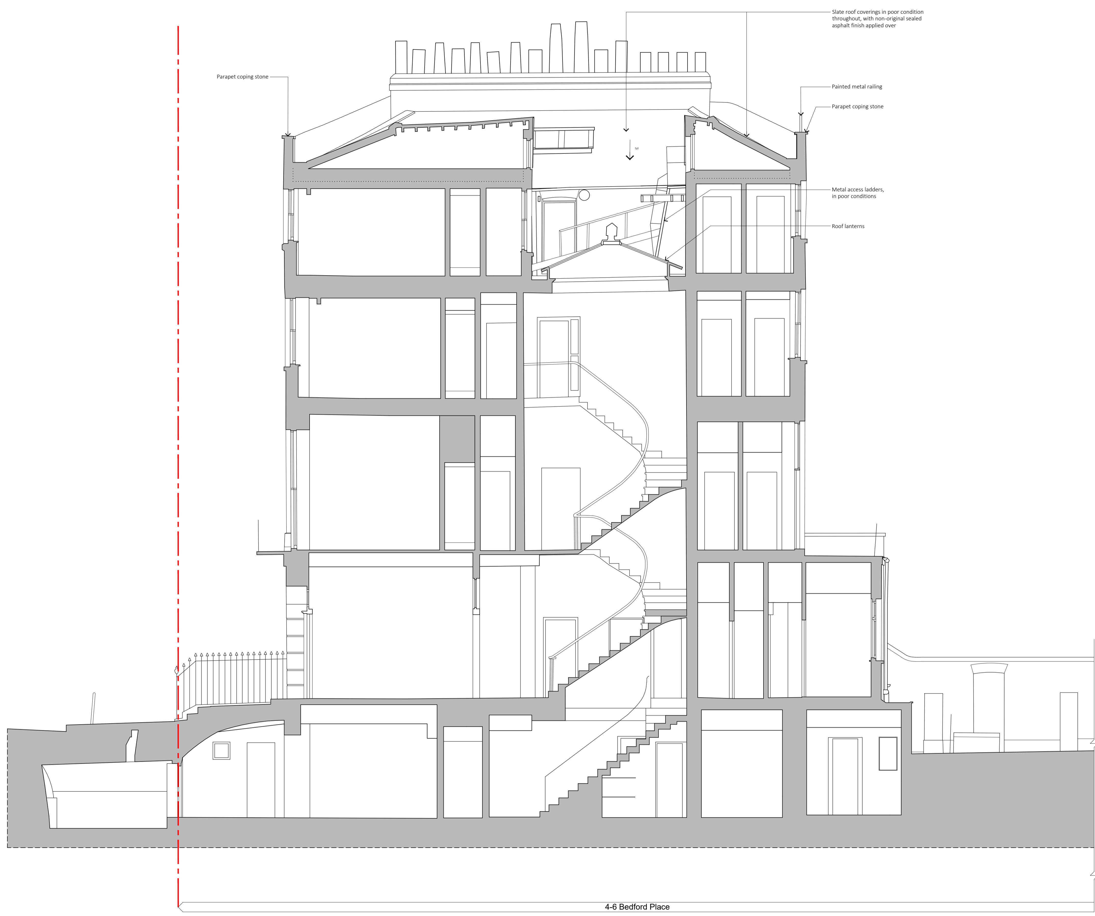
1 Existing Section A-A 1:50 @ A1
