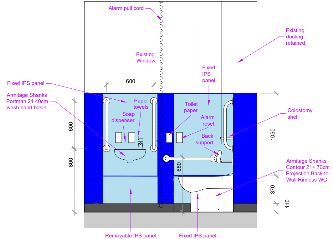
Elevation B.
