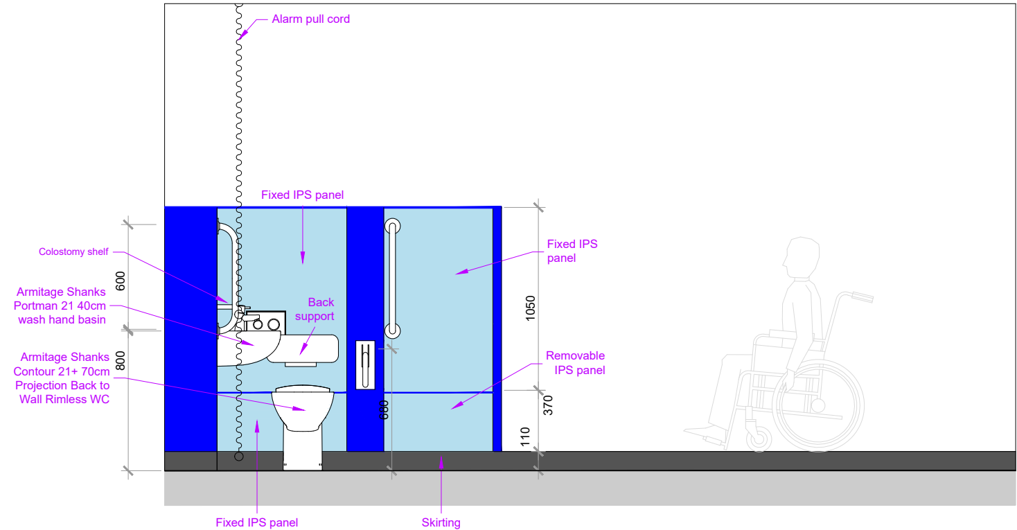
Elevation A.
