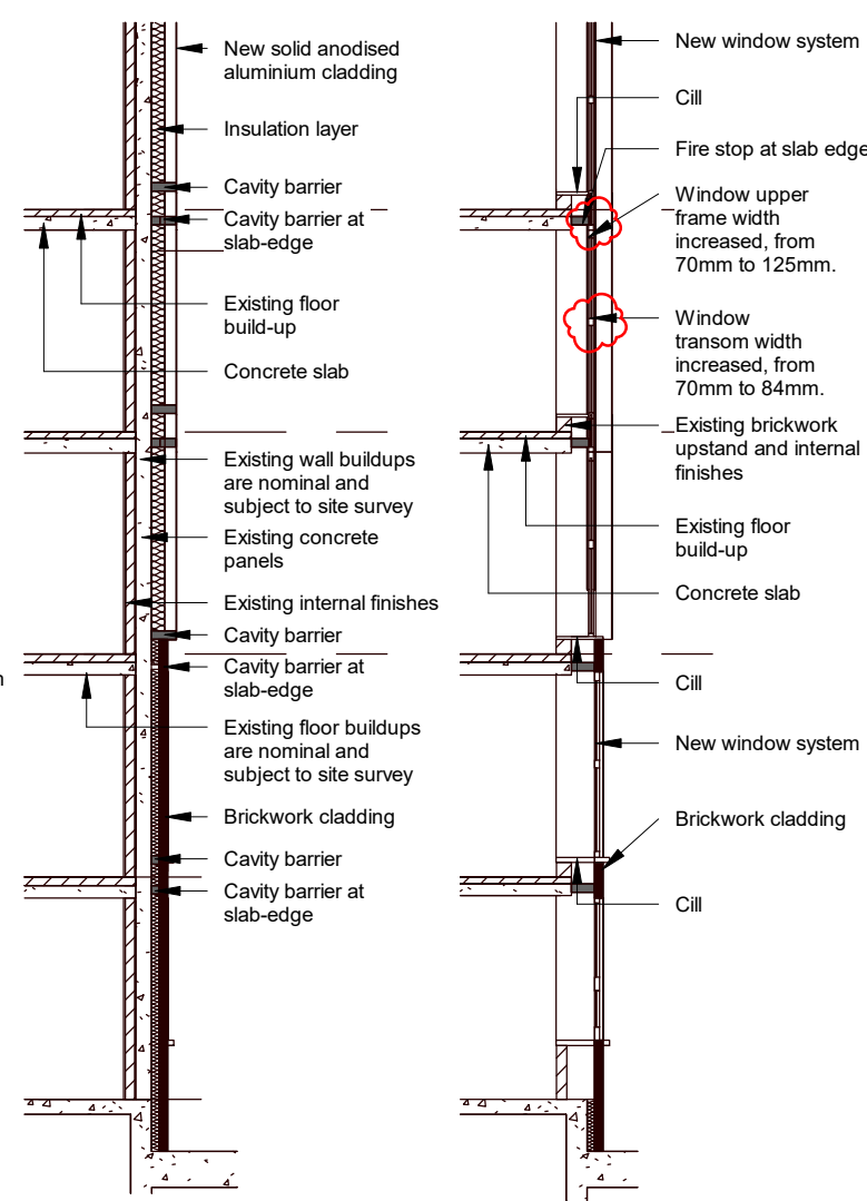
2 E3 - Detail Section 1 1 : 100
