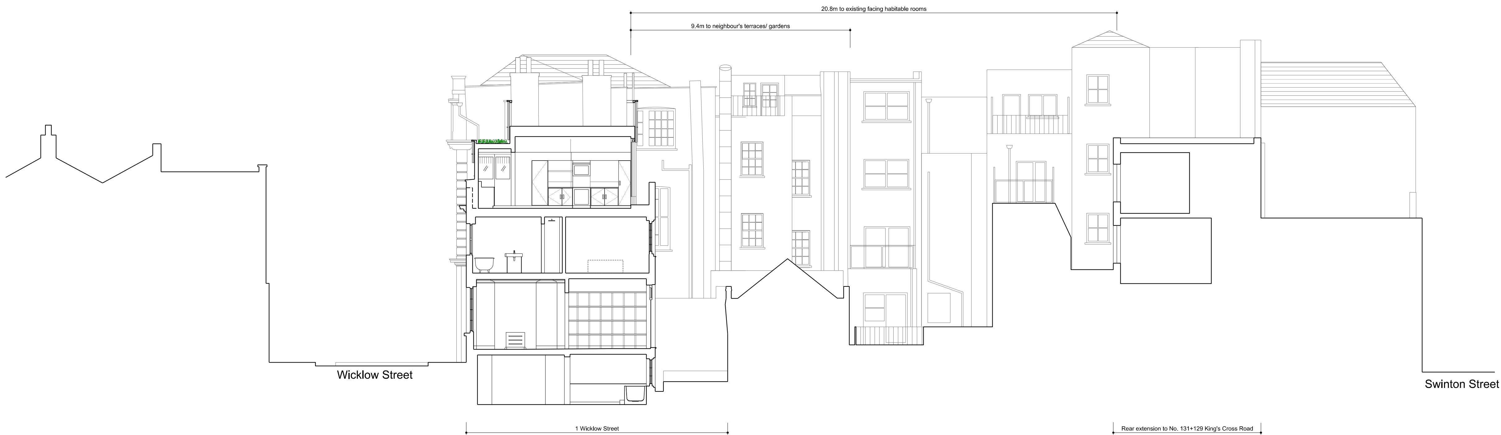
Section A-A
