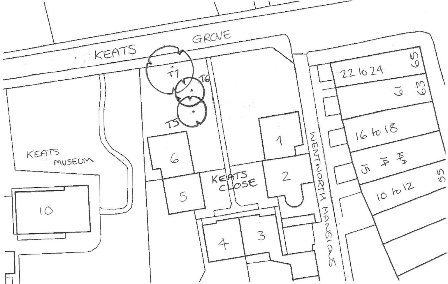
SITE PLAN FOR 6 KEATS CLOSE LONDON NW3 2RP
