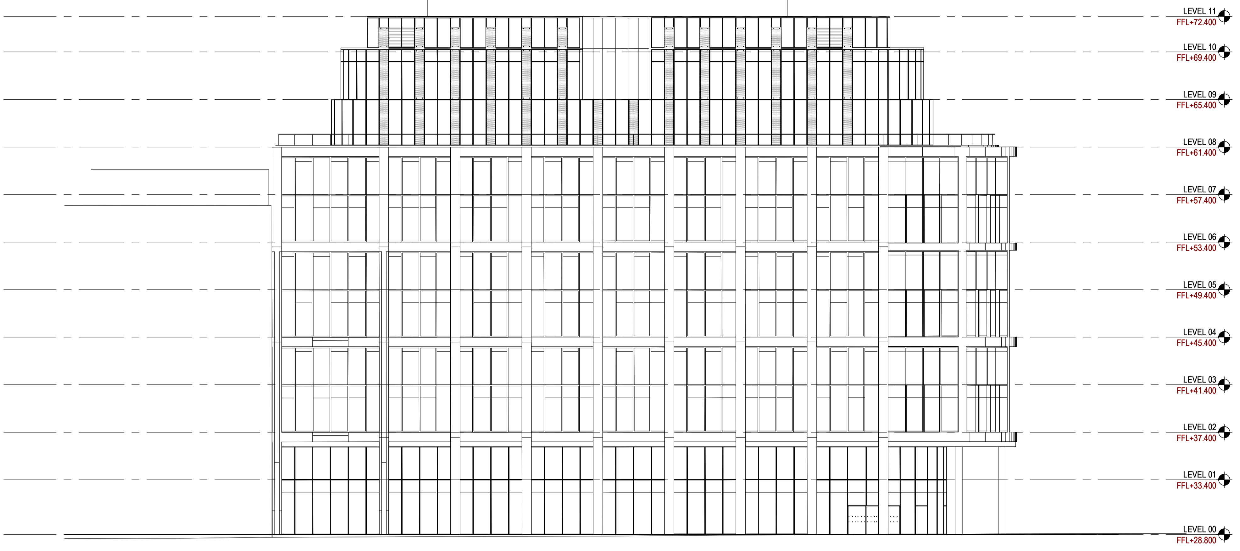
02 ELEVATION WEST_EXISTING SCALE: 1 : 200
