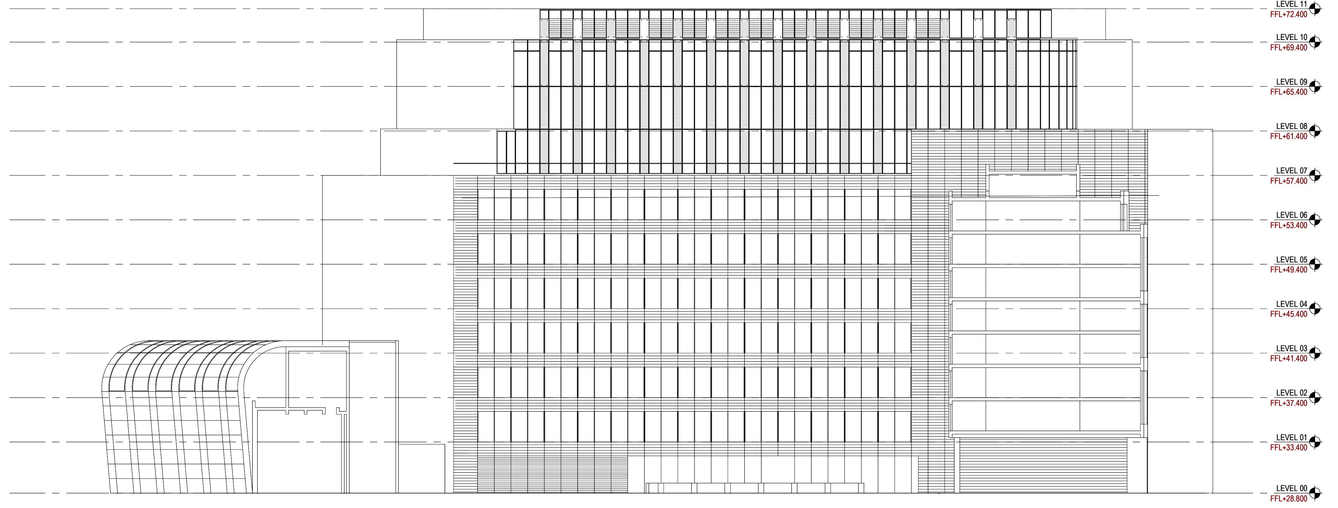
02 ELEVATION NORTH_EXISTING SCALE: 1:200
