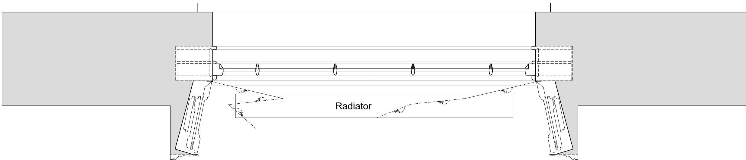
Plan Section B-B Scale: 1:10
