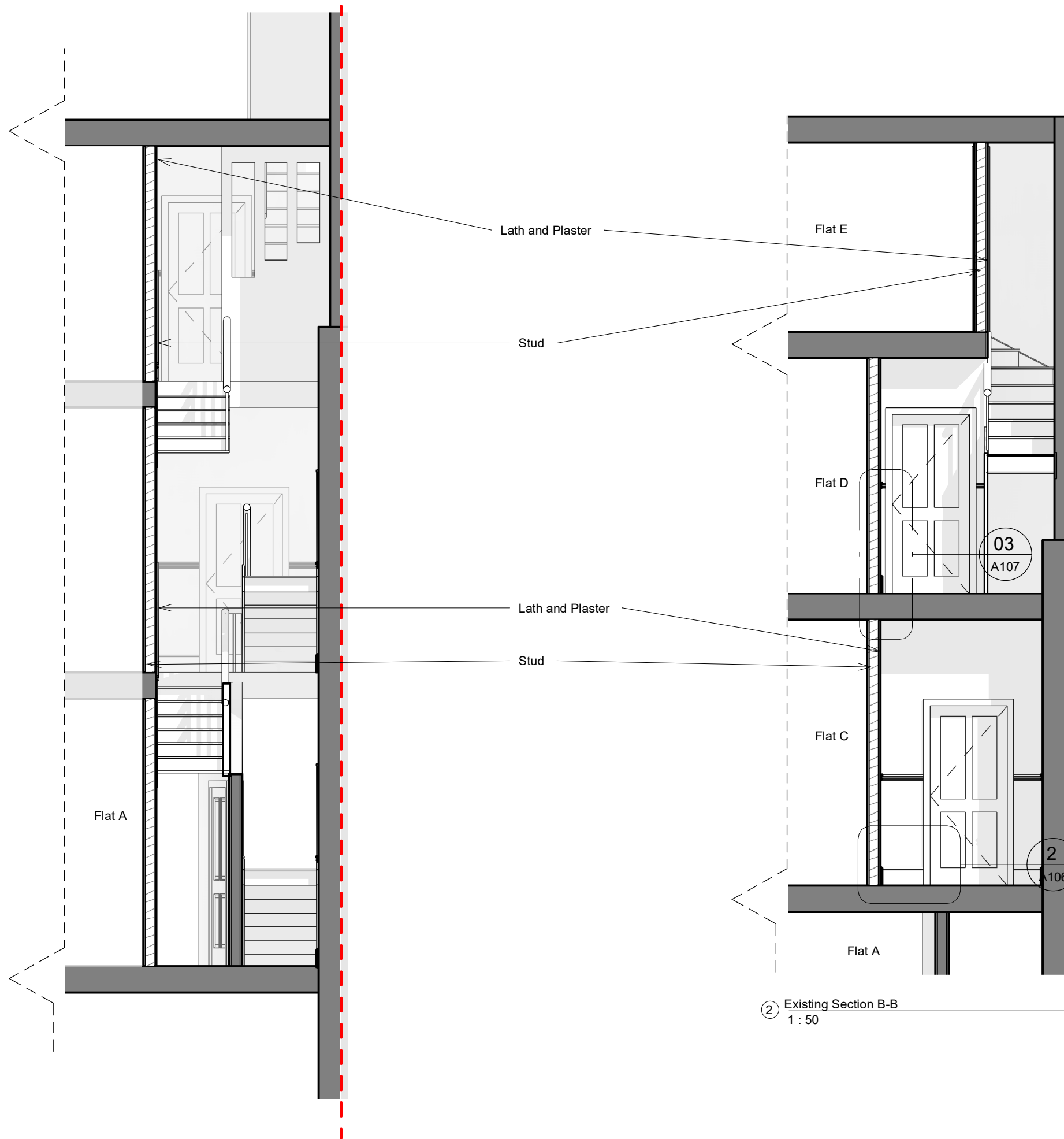
① Existing Section A-A 1 : 50
