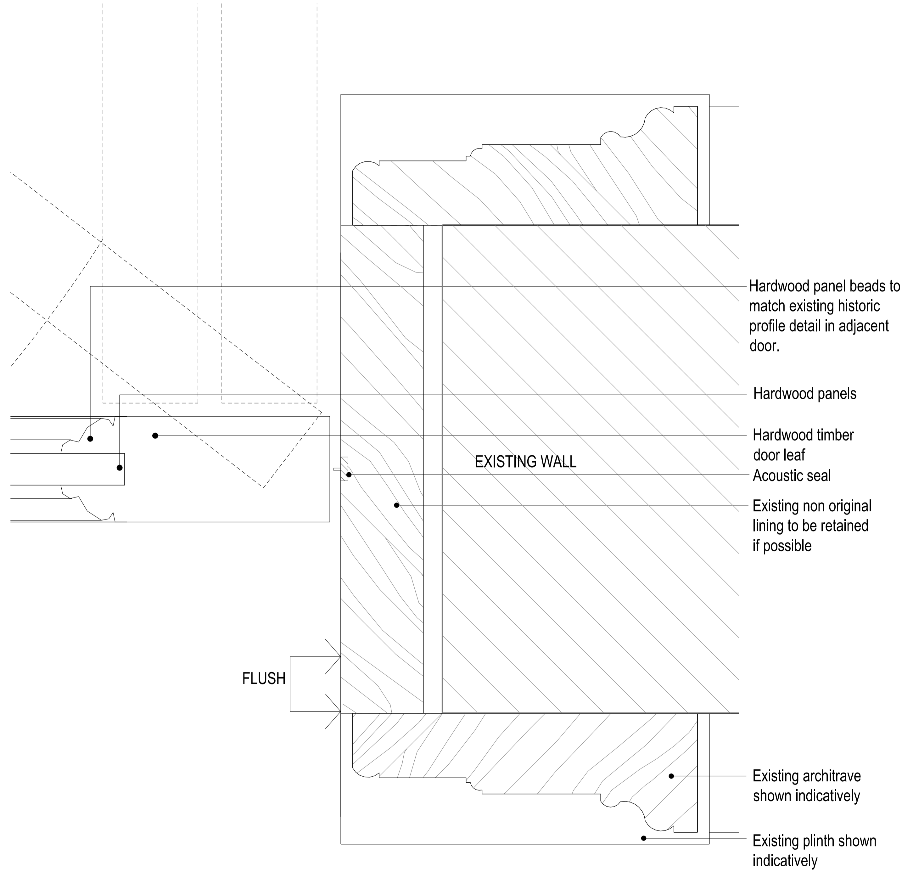
01 JAMB DETAIL scale 1:1
