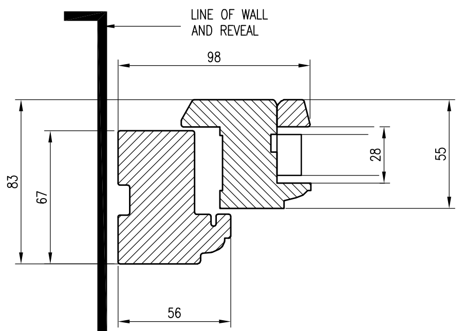
JAMB SECTION SCALE 1:2
