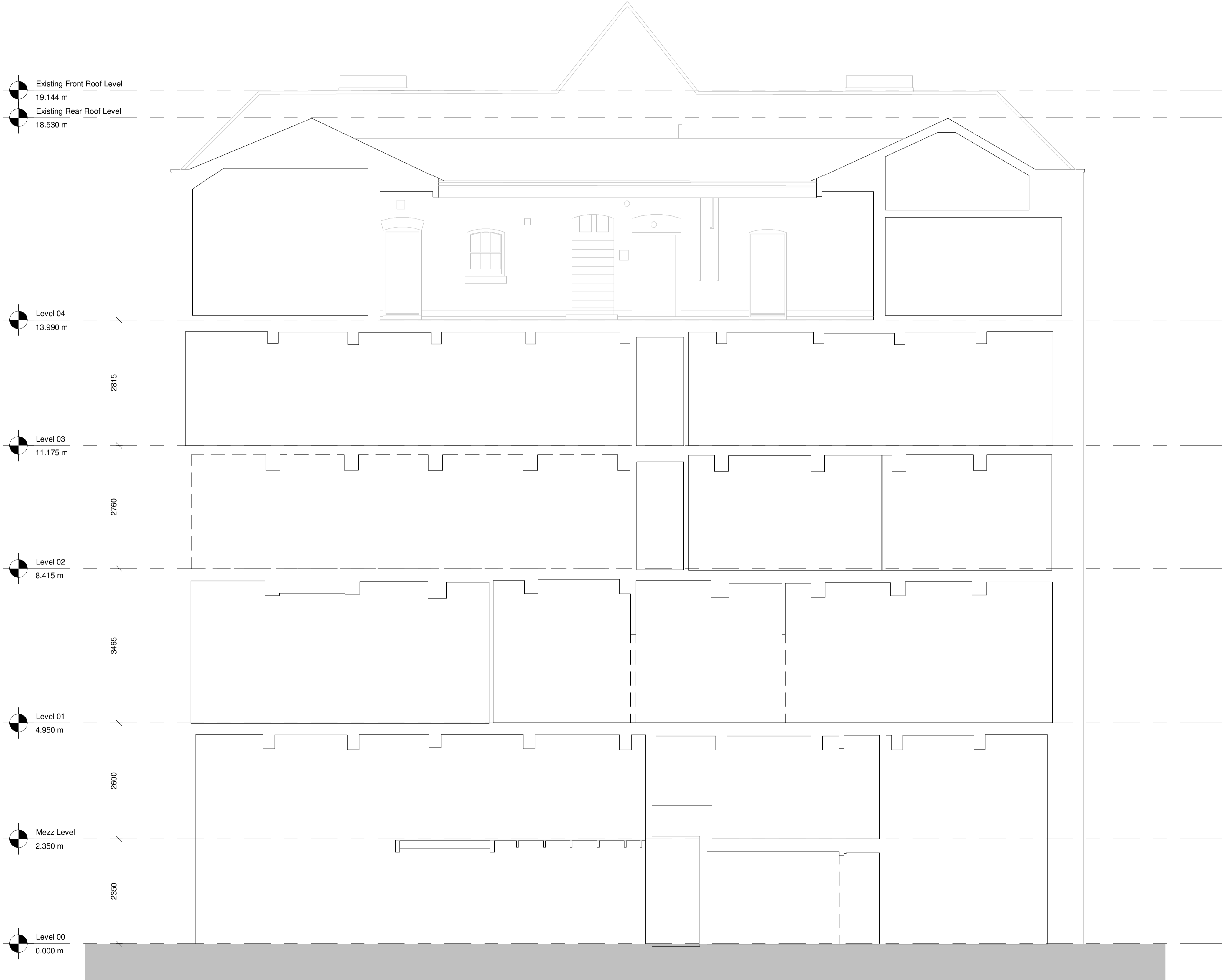
1 Section DD - Existing 1 : 50
