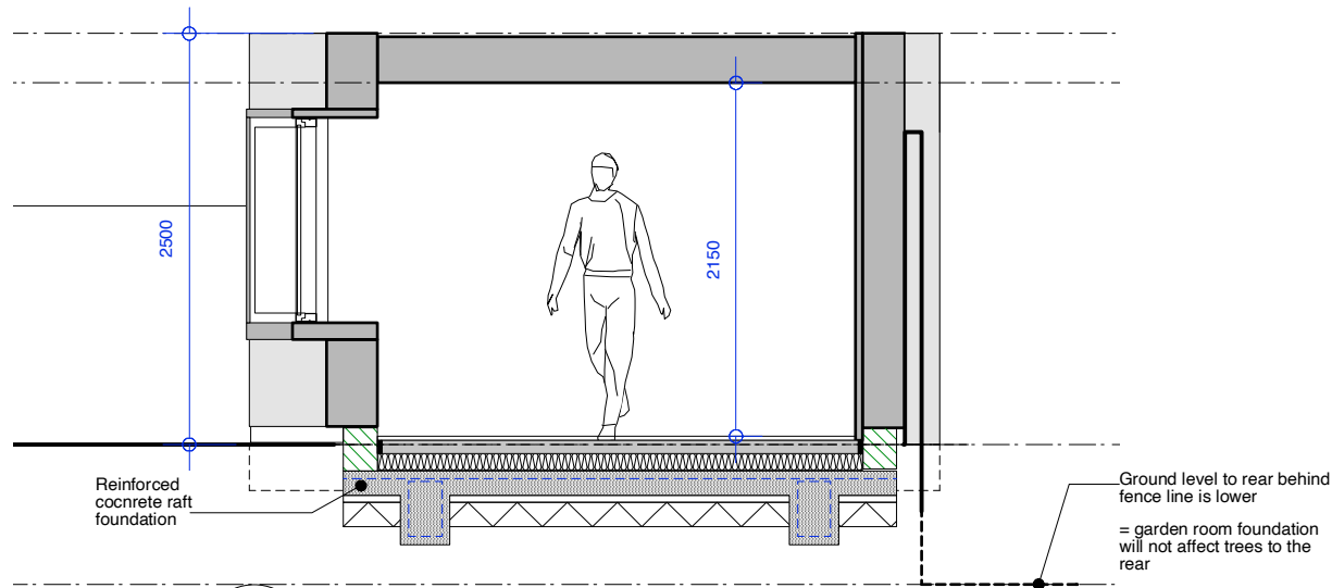
3 Section AA Scale: 1:50
