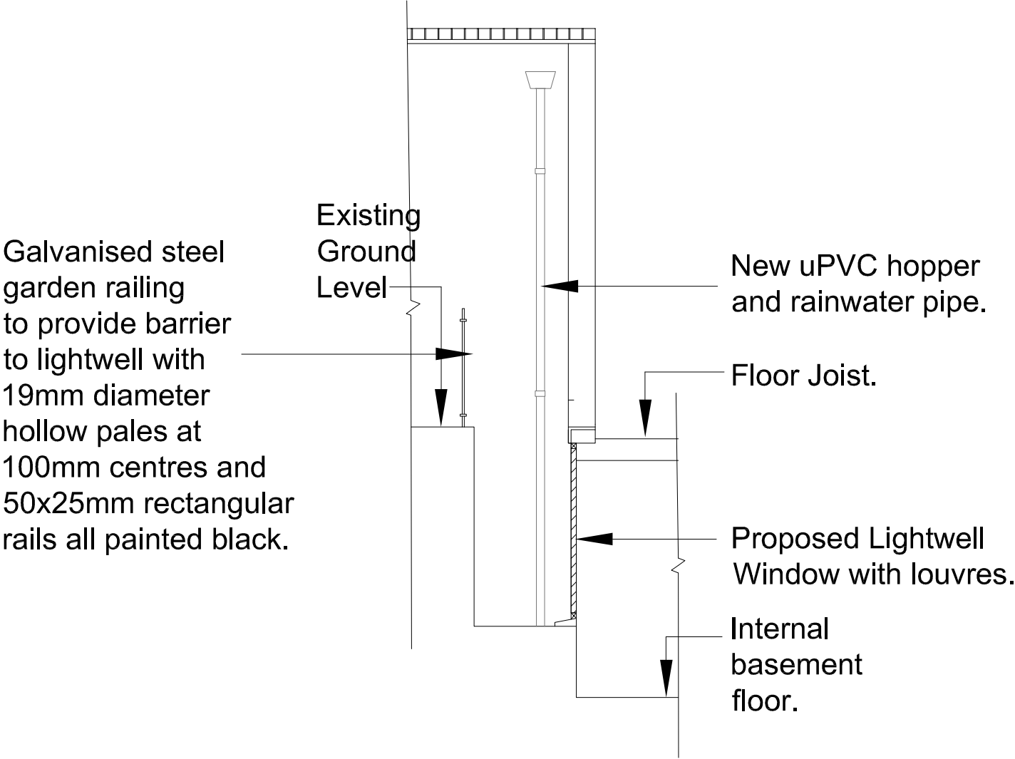
SECTION A-A
