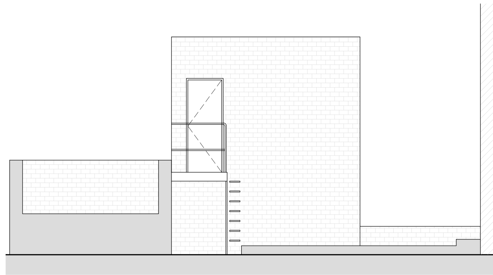
A SECTION A Scale: 1:50@A1
