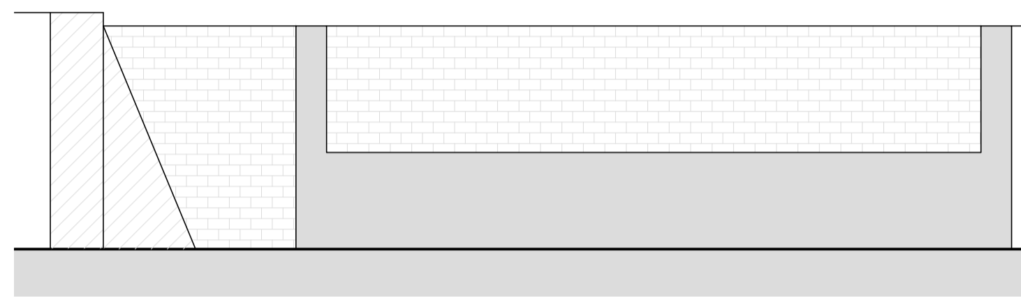
B SECTION B Scale: 1:50@A1
