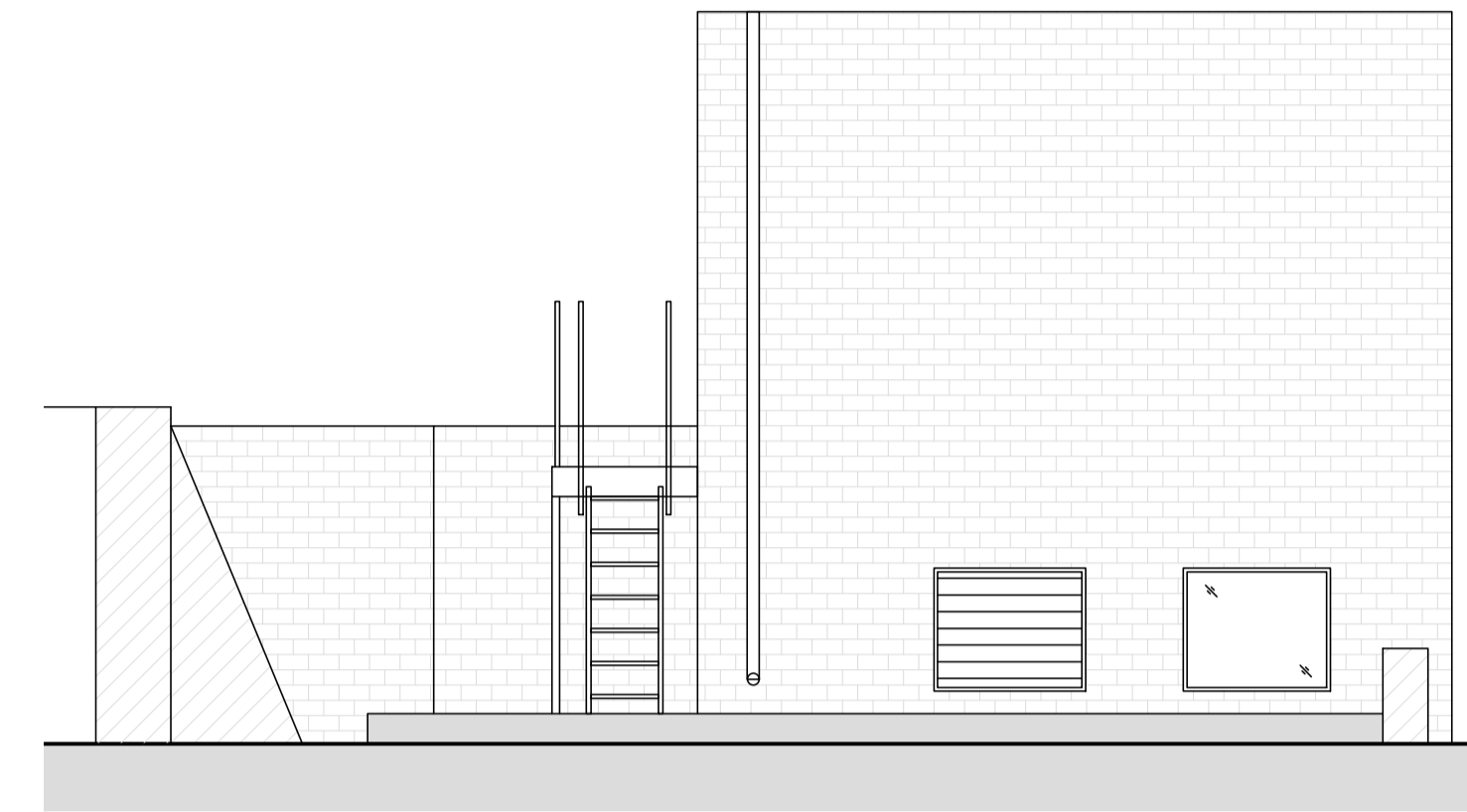
C SECTION C Scale: 1:50@A1
