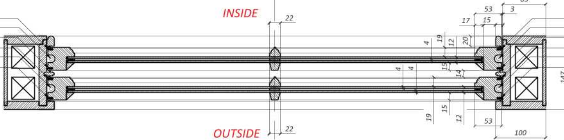
PLAN A-A 12 MM DGU
