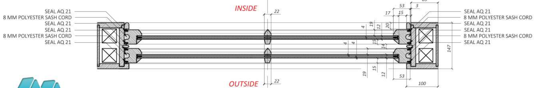
PLAN A-A 12 MM DGU
