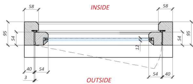
PLAN A-A 12 MM DGU
