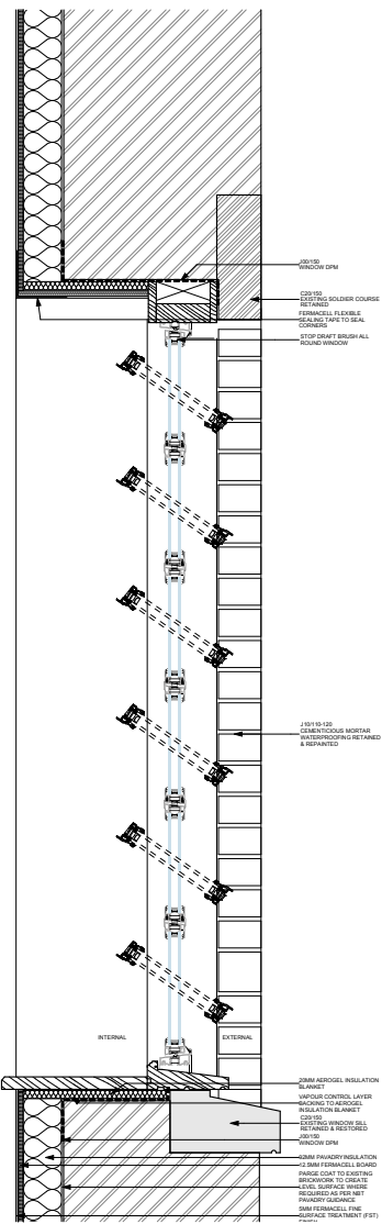
Section A-A
