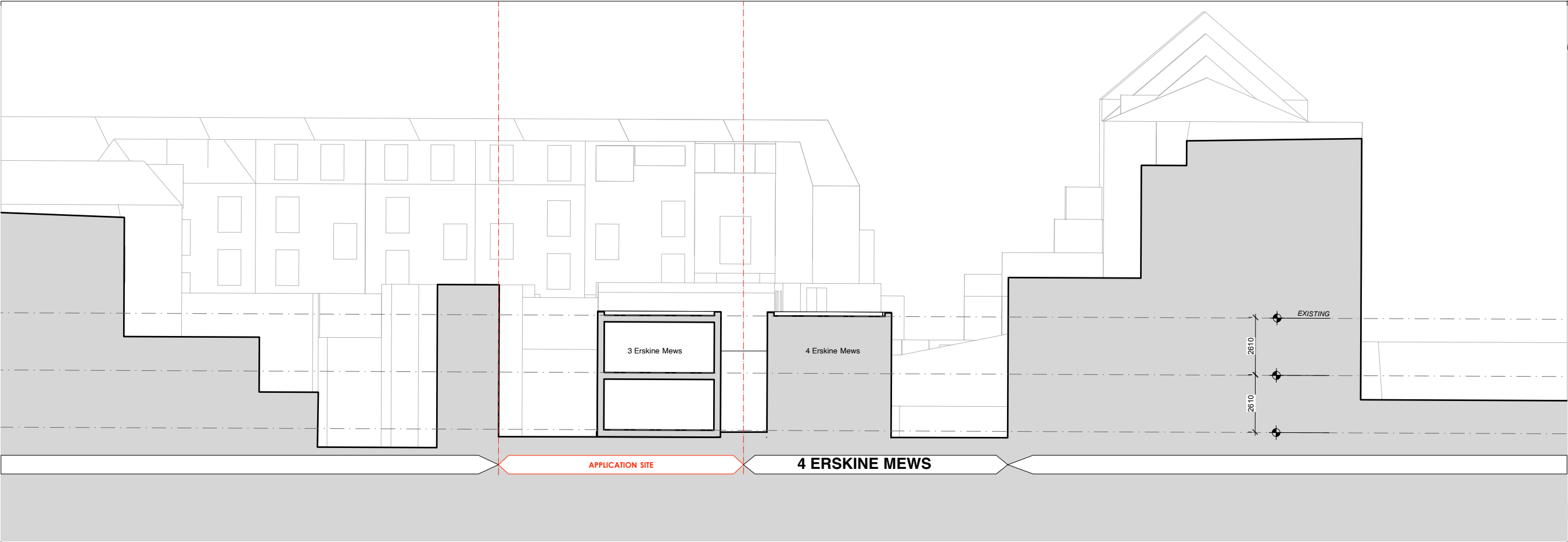
01 Existing Section C-C ES.02 1:100 @ A1 | 1:200 @ A3
